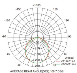
Distribución lumínica
